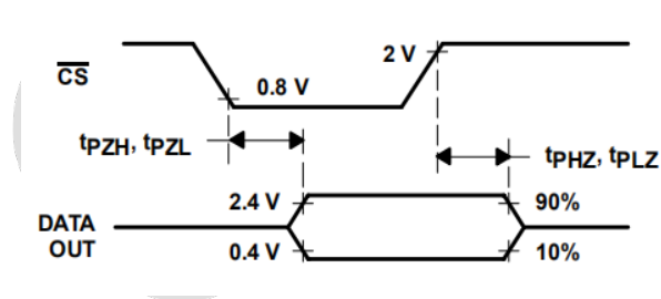
图3.数据输出到Hi-Z电压波形
