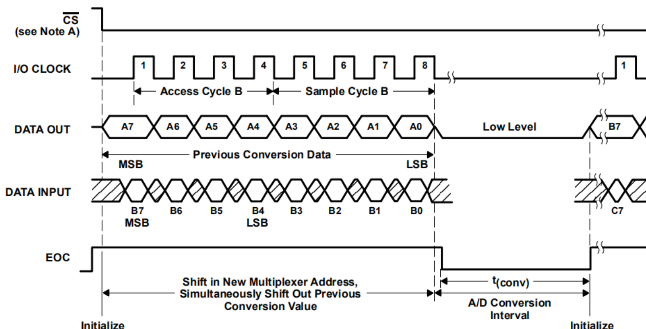
图11.首先使用MSB进行8时钟传输的时序
