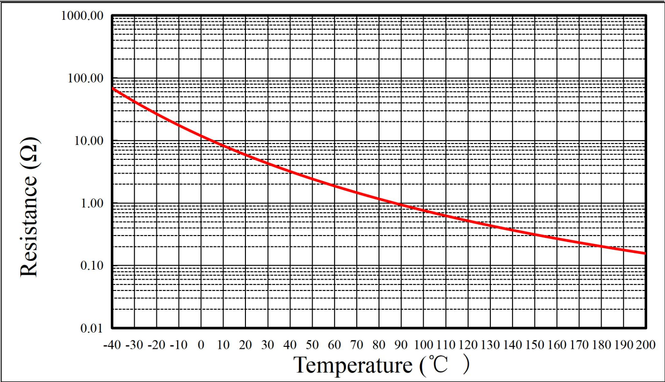
9.1.1 R-T chart 阻温特性表
