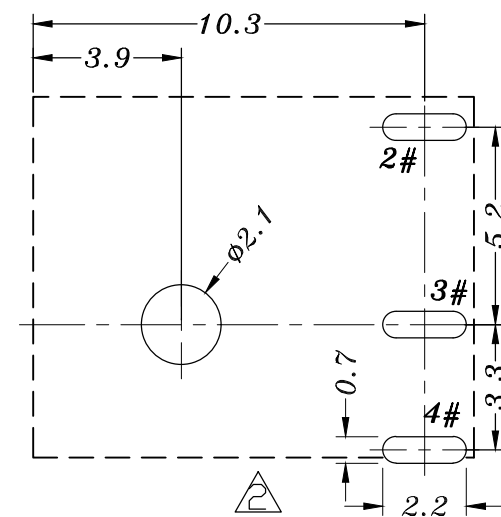
P.C.B LAYOUT
