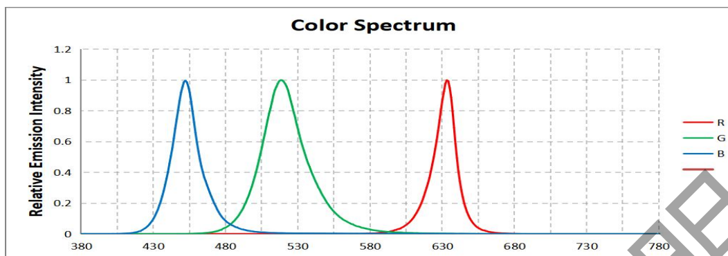
■ 光谱图, T_a=25^{\circ}\text{C}
