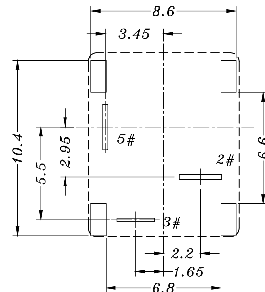
P.C.B LAYOUT
