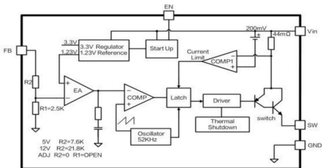
图3. 2575 方框图
