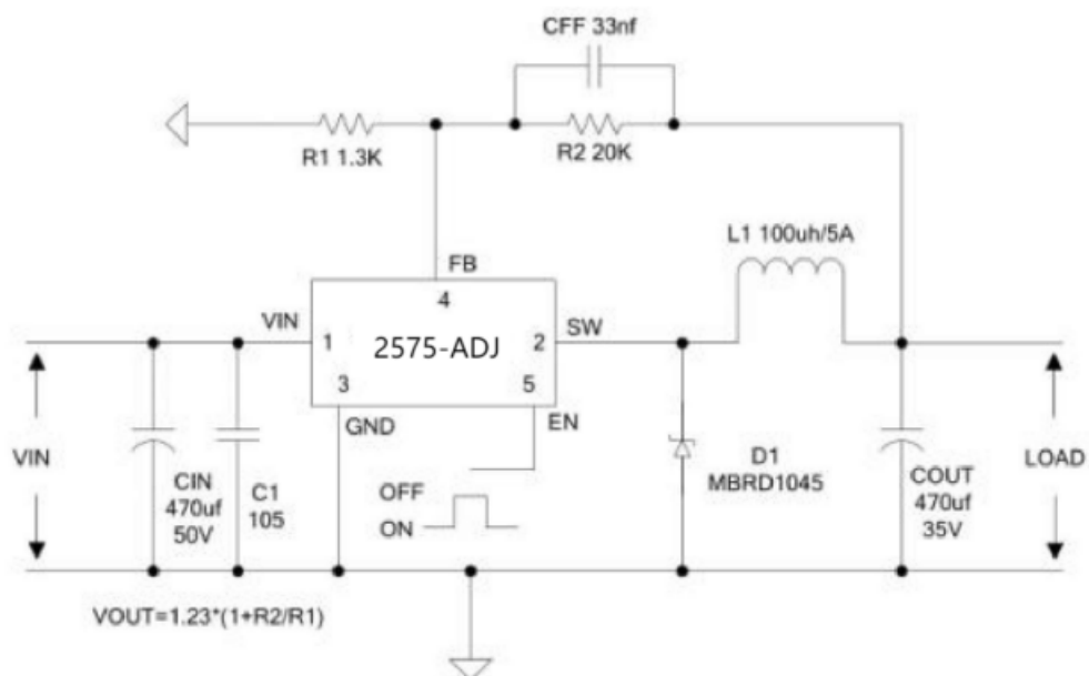
图 9. 2575-ADJ 大功率应用电路图 ( V_{IN}=24V, V_{OUT}=20V, I_{OUT}=2.5A )
