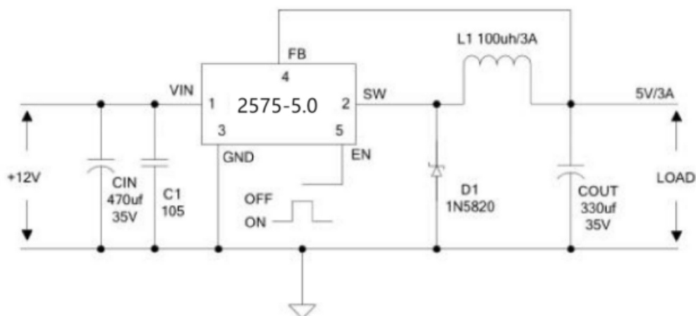
图4. 2575 系统参数测量电路(12V-5V/3A)
