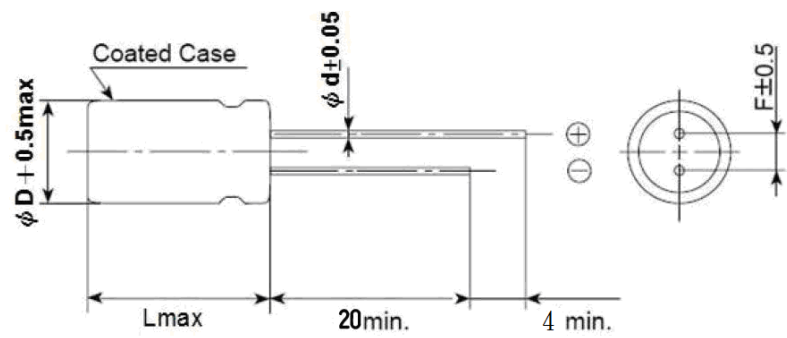
Fig. 2 Dimension Table 7 Dimension
