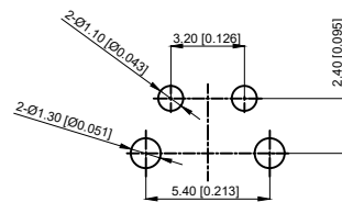
安装位置图
