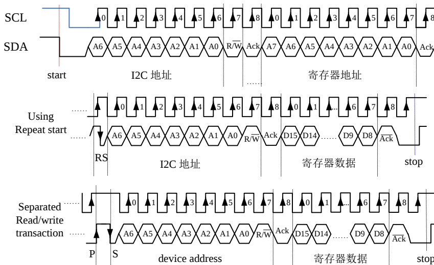
图6 AW9136 I²C 接口读操作时序
