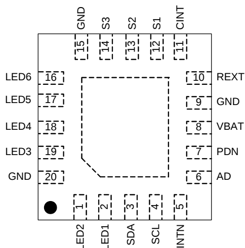
AW9136引脚俯视图
