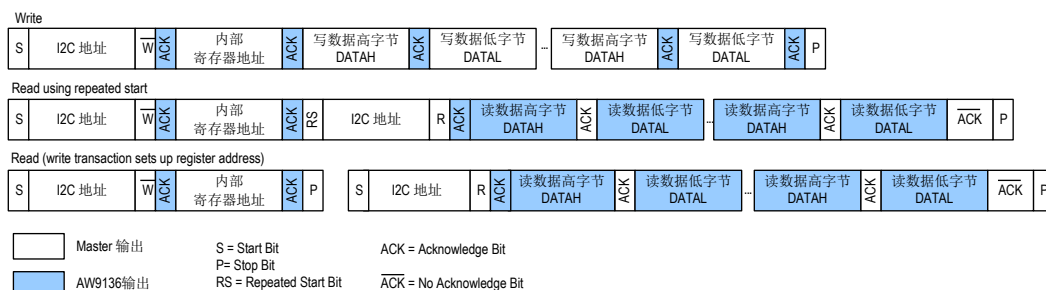
图7 AW9136 I²C 接口写、读操作数据传输格式
