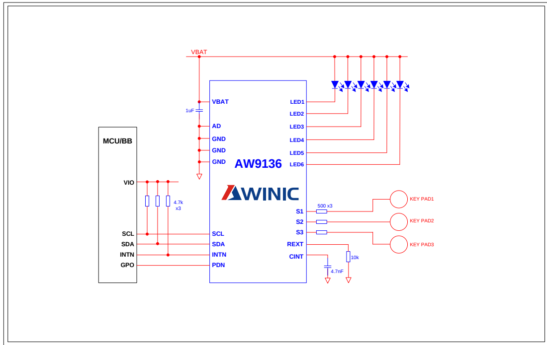
图2 AW9136 典型应用图
