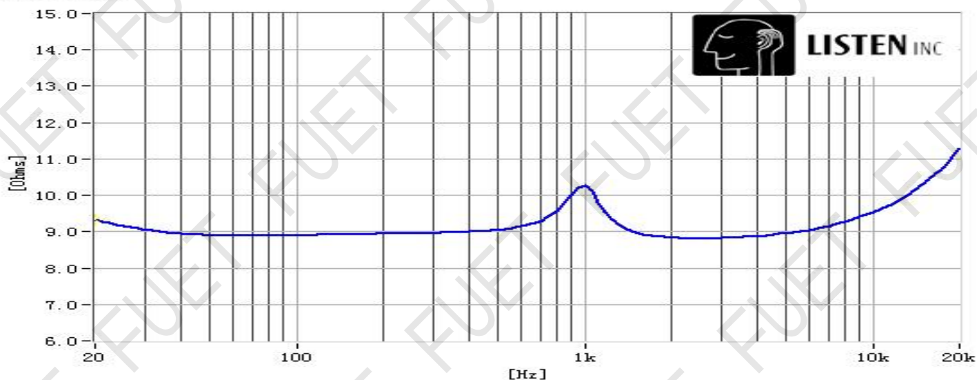
阻抗曲线
