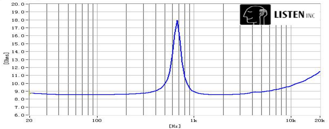
阻抗曲线
