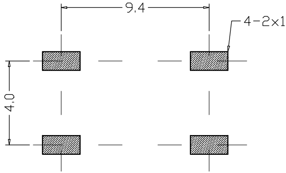
PCB线路板图
