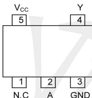
SOT353
