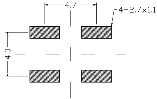
PCB线路板图
