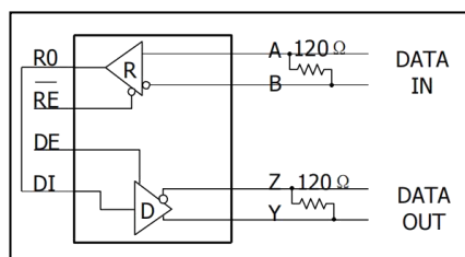
图 11. SN65HVD3080/ SN65HVD3083/ SN65HVD3086 全双工模式下的中继器
