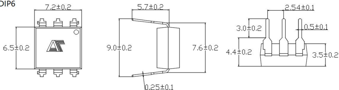
DIP6-M
