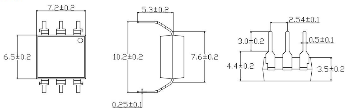
SMD6
