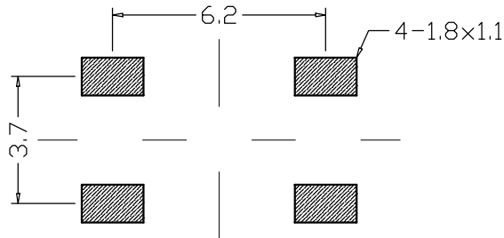
PCB线路板图
