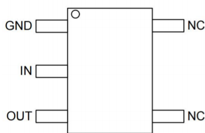
SOT23-5
