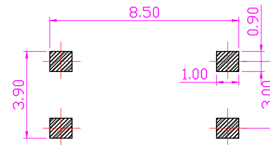
PCB. 焊接图
