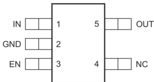
SOT23-5
