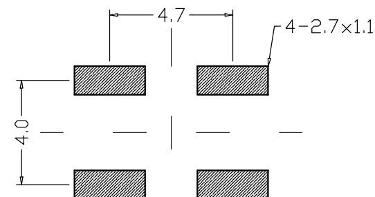
PCB线路板图
