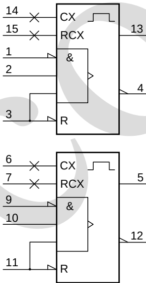
图 2 IEC 逻辑符号
