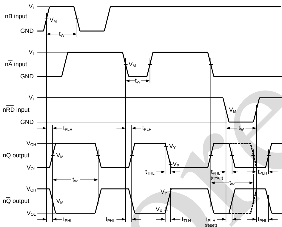
图6 输入 (nA, nB, nRD) 到输出 (nQ, nQ) 的传输延时和输出转换时间
