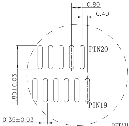
DETAIL B(SCALE 2:1)
