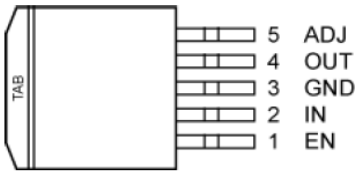
引脚排列（顶视）
