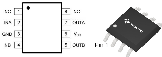
SOP-8 顶视图
