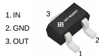
SOT-323
