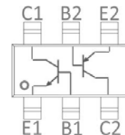
SOT-363
