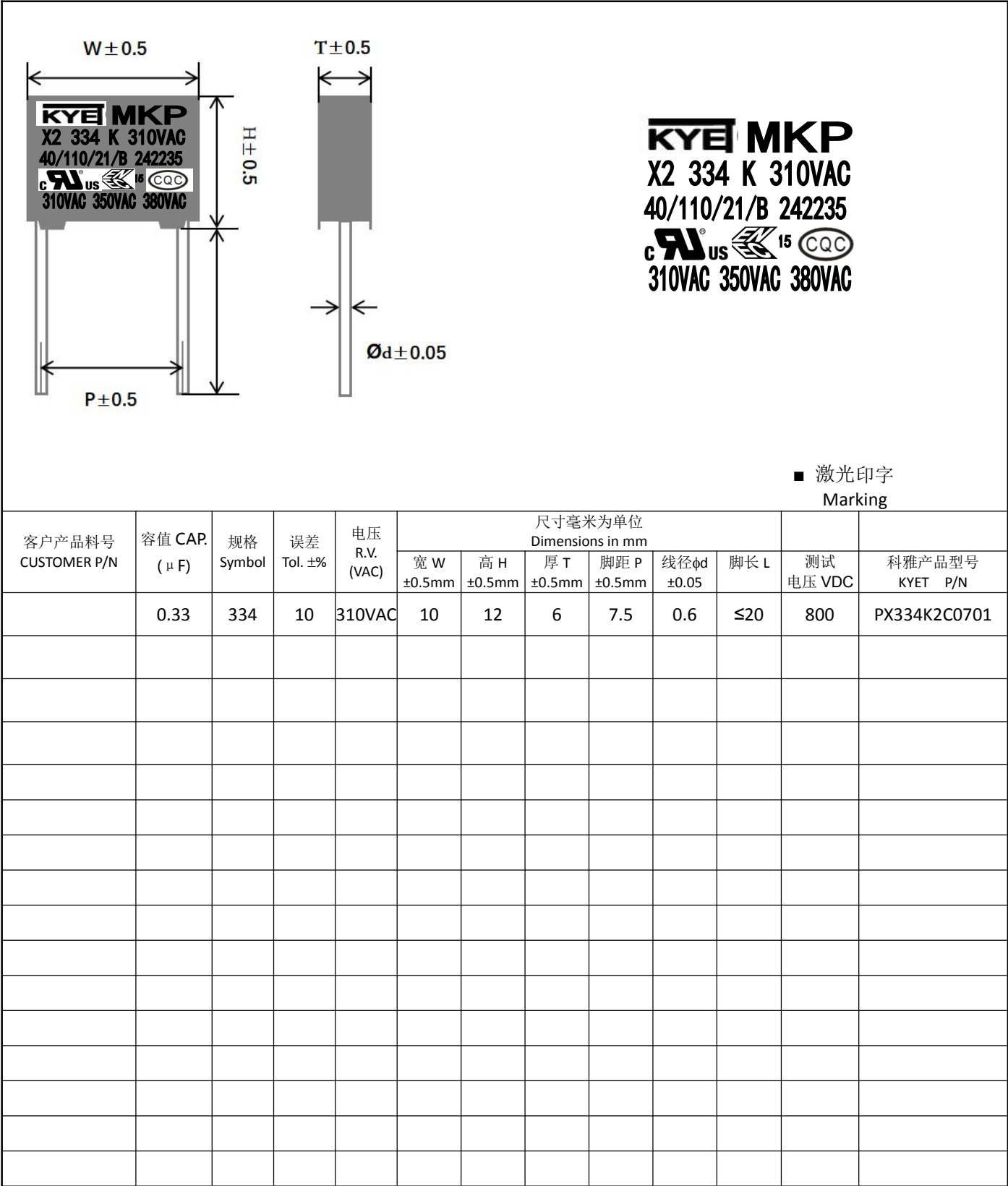
产品尺寸图 PRODUCT DIMENSIONS
