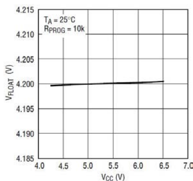
浮充电压 vs 电源电压
