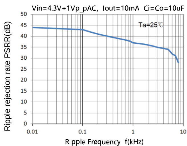
纹波抑制
