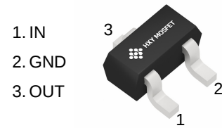
SOT-323
