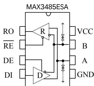
图 1 MAX3485ESA引脚分布图
