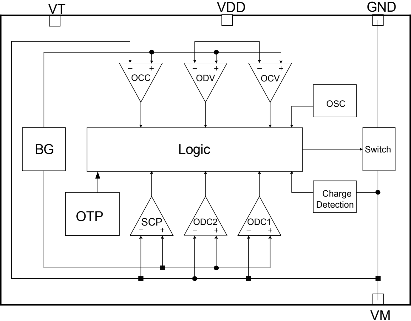
功能框图
