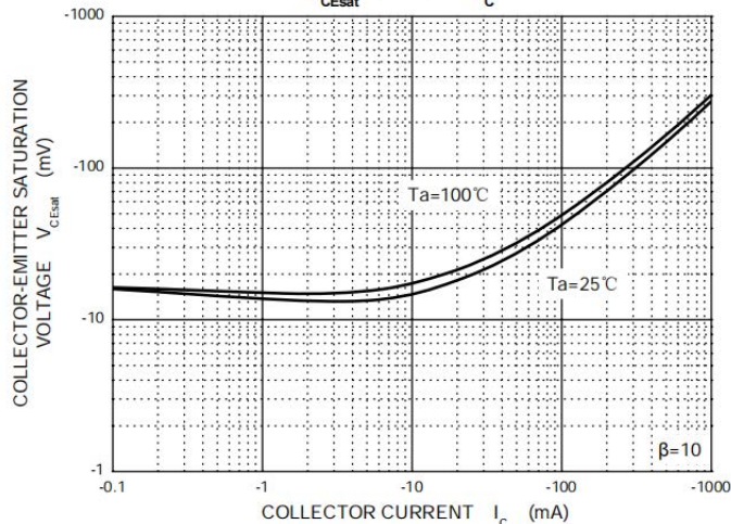
V_{CEsat} — I_c
