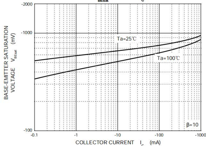
V_{BEsat} — I_c
