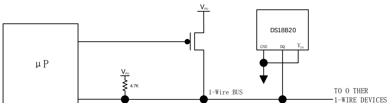
图 4. 在温度转换期间为寄生供电的 DS18B20供电
