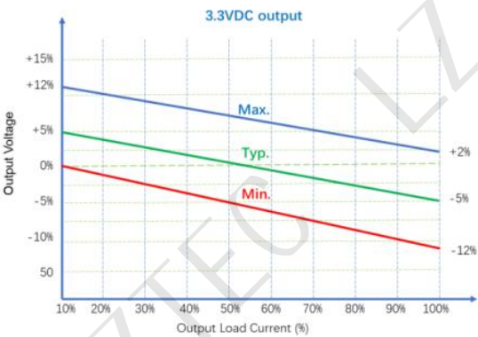
产品特性曲线图
