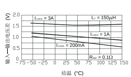
电压降落
