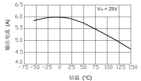
电流极限值
