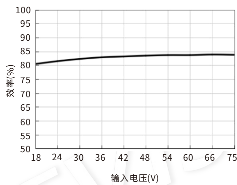
效率Vs输入电压(满载) URA4815YMD-6WR3
