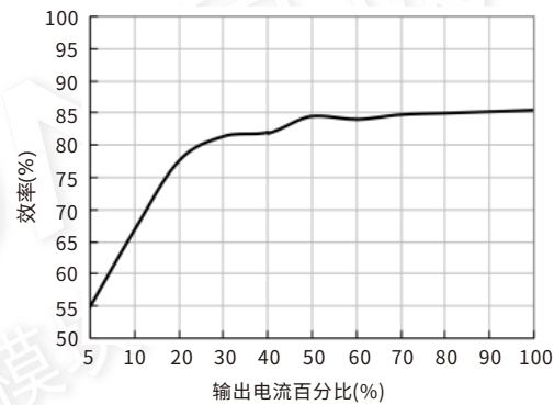
效率Vs输出负载(Vin=48V) URA4815YMD-6WR3
