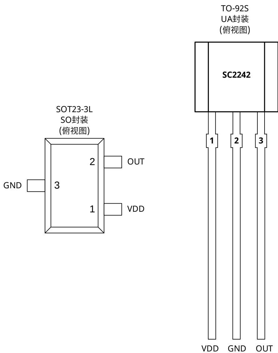
图 2 引脚描述
