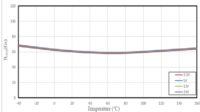
SC2443 B_{HYS} VS. Temperature
