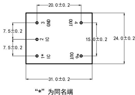
底视图
