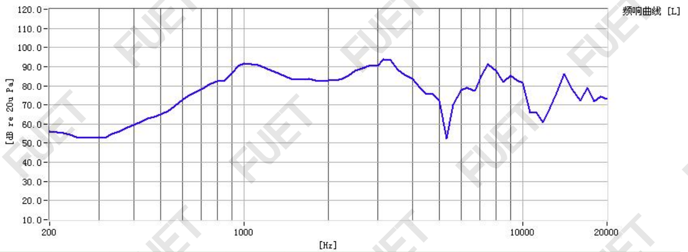
频响曲线
