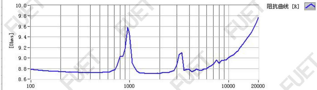
阻抗曲线
