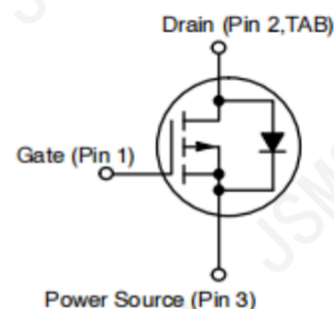
TO-263-2L
