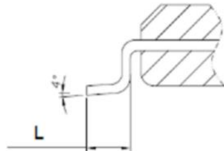
A 局部放大
