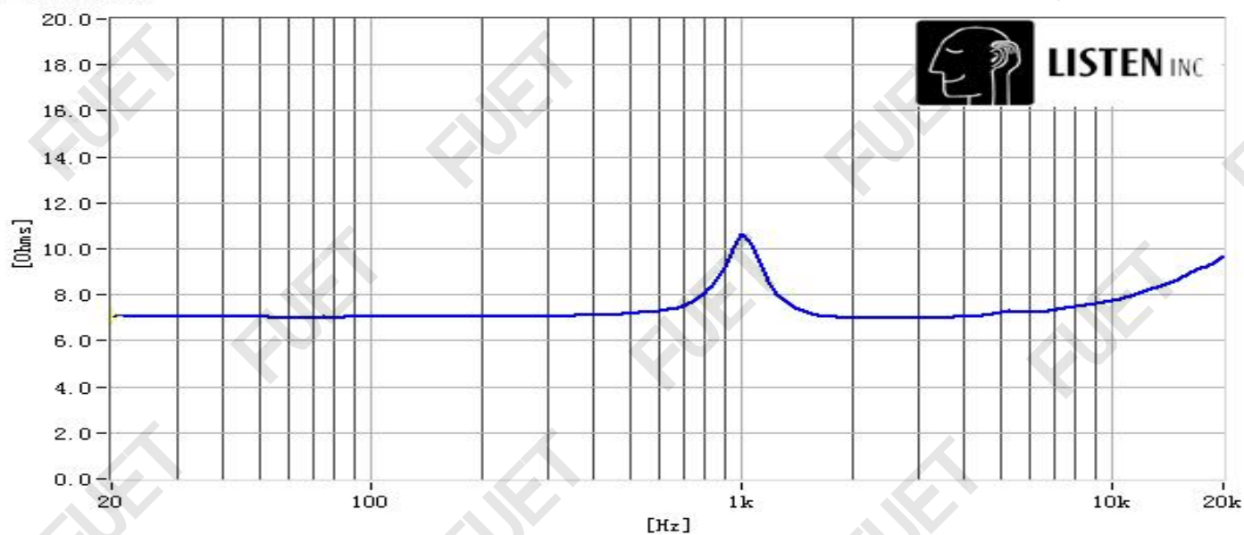
阻抗曲线
