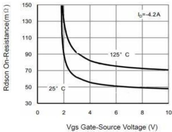
Rdson vs.Vgs
