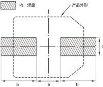
SMD推荐焊盘尺寸
