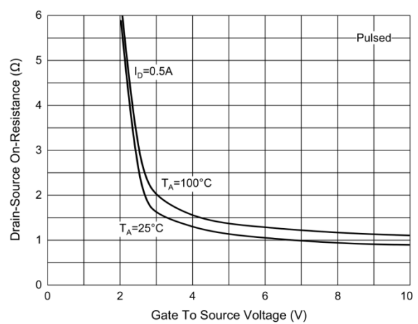
R_{DS(ON)}-V_{GS}
