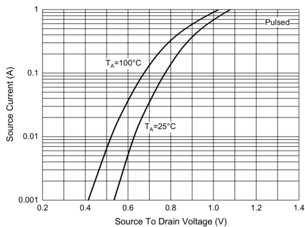
I_S-V_{SD}
