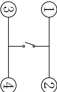
电路图
