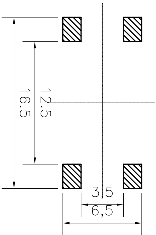
PCB. 焊接图
