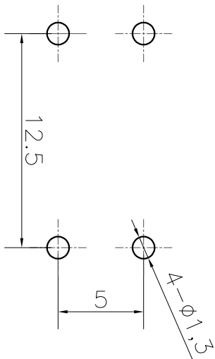
PCB. 焊接图
